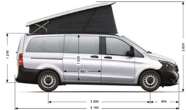
Vue latérale, toit relevable ouvert
