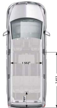
Banquette en position siège
