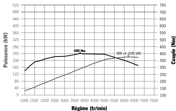
Moteur V6
