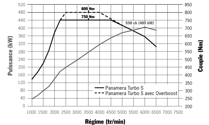
Moteur V8 biturbo de la Panamera Turbo S
