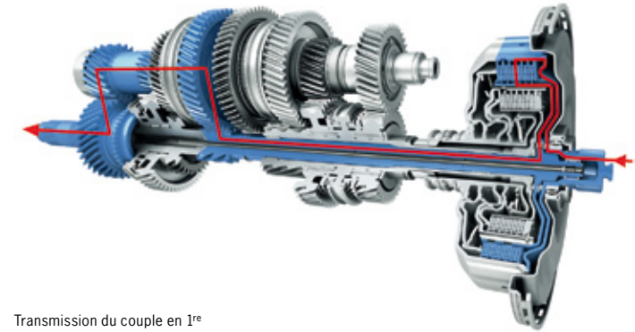
Transmission du couple en 1 e
