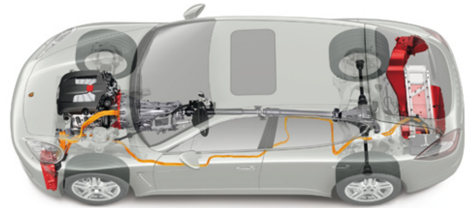
Système Parallèle-Full-Hybrid
