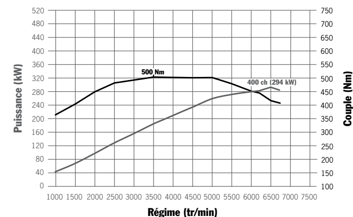
Moteur V8
