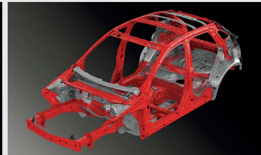
STRUCTURE DE CAISSE LÉGÈRE ET RIGIDE POUR AMÉLIORER LA SÉCURITÉ PASSIVE
