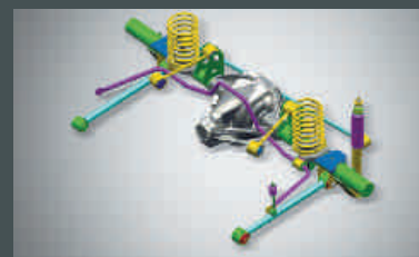
Suspension arrière à cinq bras.
