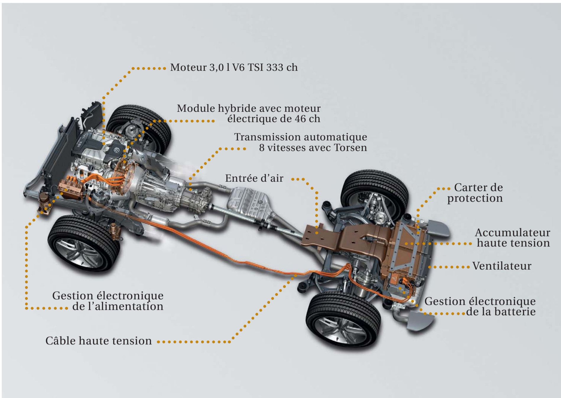
Schéma de la motorisation hybride
