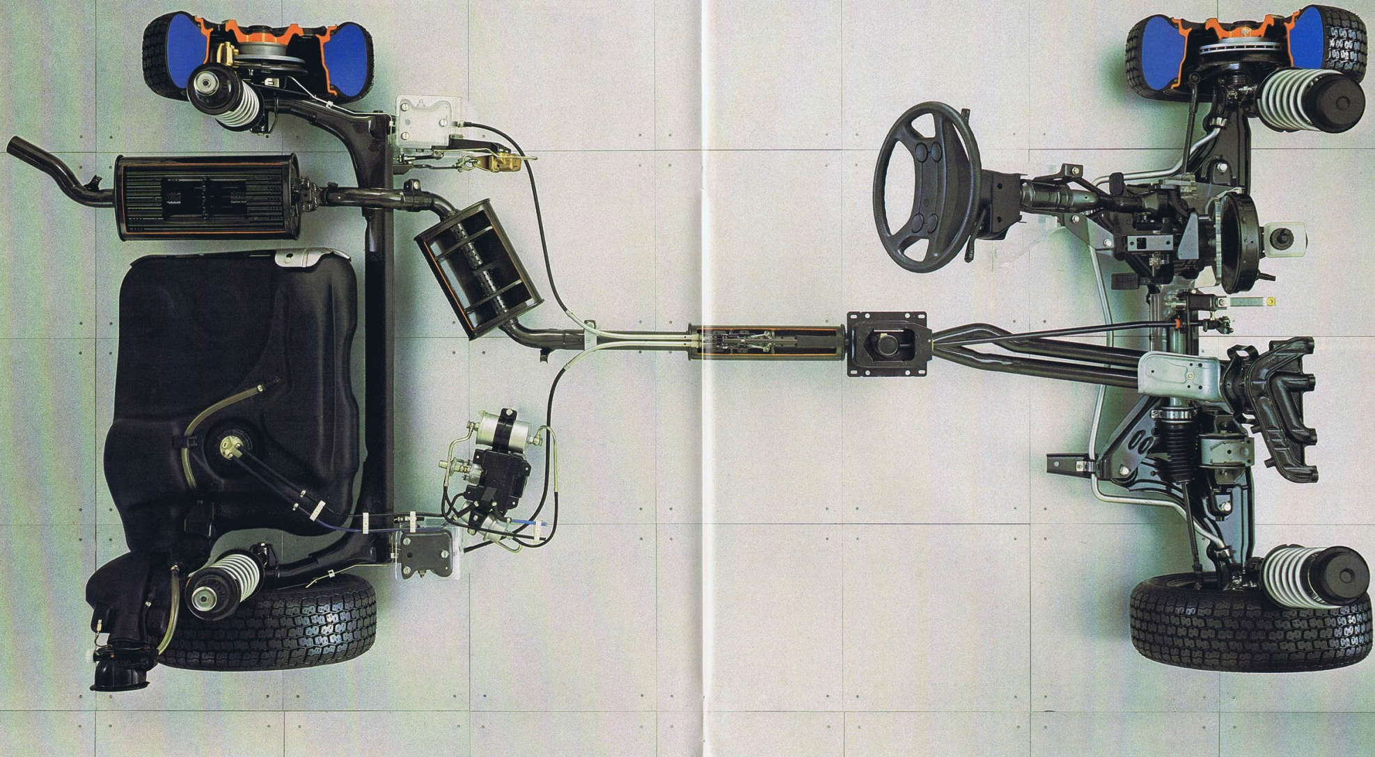
Trains de roulement de la GTI.
