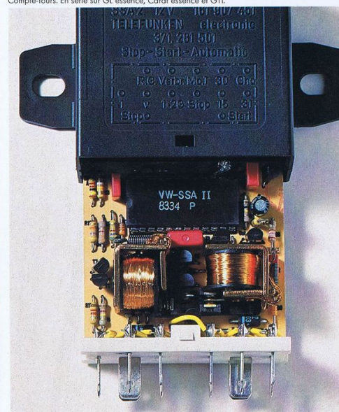
Système économiseur d'essence stop-start.
