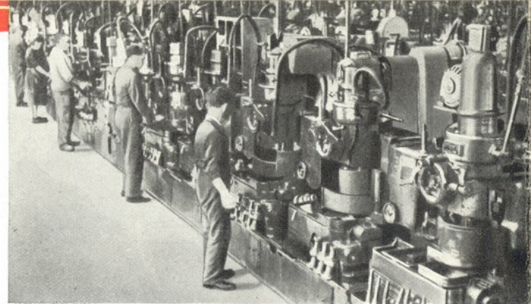
La chaîne de taillage des pignons
