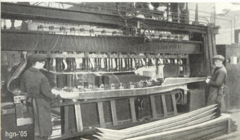
Machine à souder électriquement les longerons
