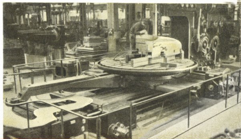
Machine à reproduire les matrices d'emboutissage
