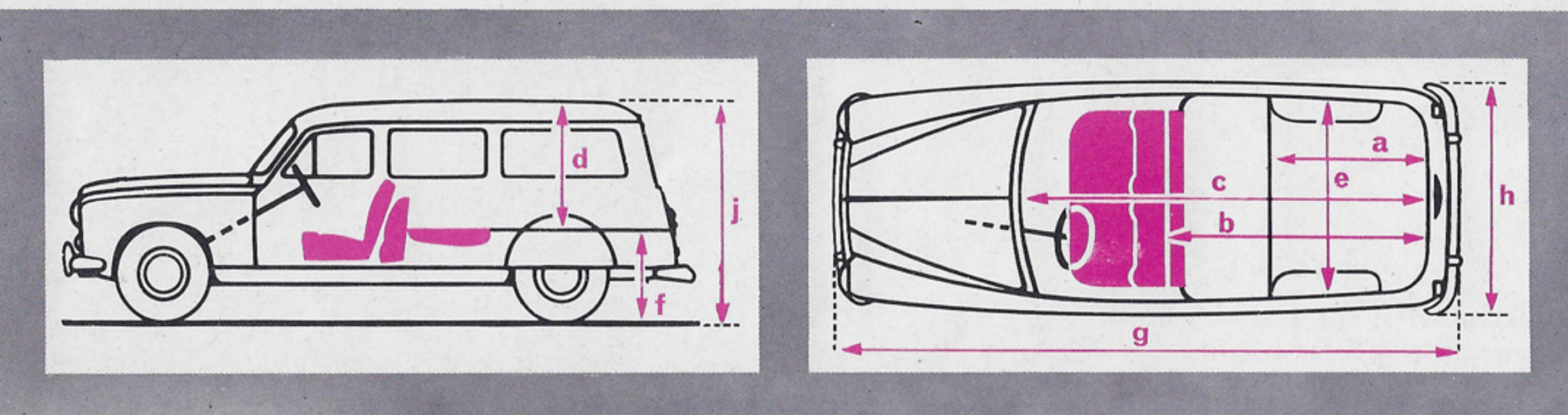
Conducteur et 1 ou 2 passagers : grand volume et vaste surface utiles pour le transport des marchandises.
