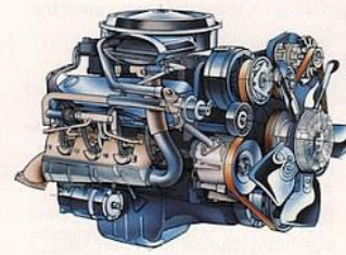
7.4L V8
