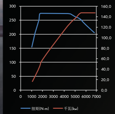
THP 200 发动机的功率扭矩图
