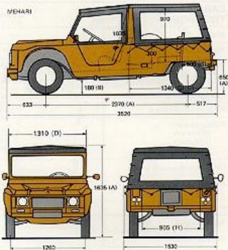
A: à vide D: largeur aux bandeaux H: entrée de porte B: en charge G: longueur au plancher Q: banquette AR rabattue
