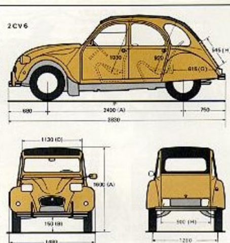
A: à vide B: en charge D: largeur aux bandeaux G: longueur du plancher H: entrée de porte
