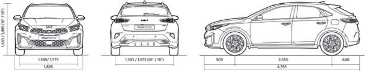
Dimensions versions Thermiques (mm)
