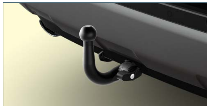
Crochet d'attelage amovible No d'art. Z3000-66340-000 No d'art. Z3000-75420-300 Prise électrique 7 broches No d'art. Z3000-75420-400 Prise électrique 13 broches
