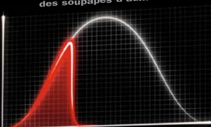
Fermeture précoce des soupapes d'admission
