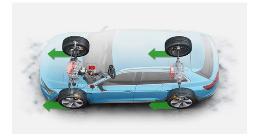
Transmission intégrale "e-quattro" [1X1]
