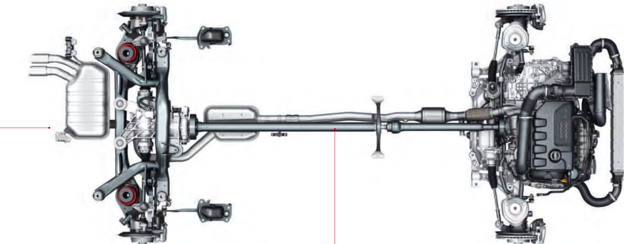
La chaîne cinématique quattro®
