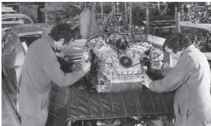
> Atelier de Fabrication moteur – Dieppe – 1976
