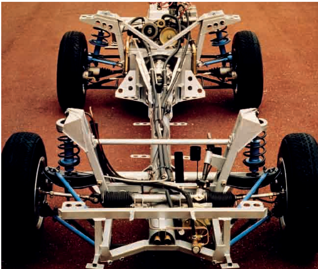
> A110 Berlinette – Châssis nu – 1975
