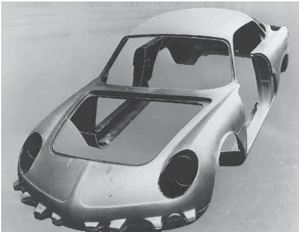
> A 110 – Coque carrosserie plastique – 1968
