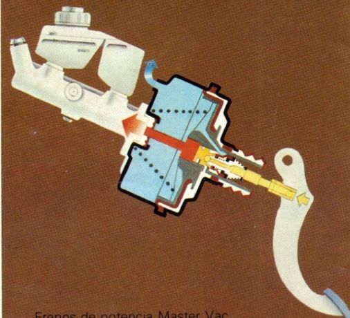
Frenos de potencia Master Vac. Equipo de fábrica en la Gama Renault 12.
