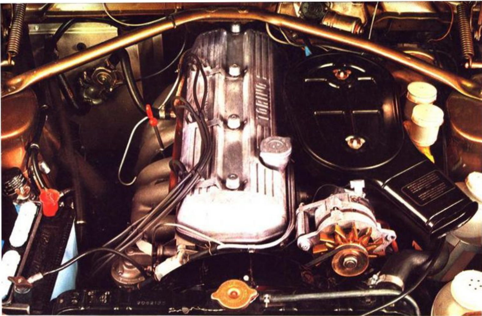
Motor Torino 7 bancadas.
