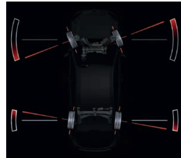
Gegensinniges Einschlagen der Hinterachse für Wendigkeit und Agilität bei niedrigeren Geschwindigkeiten
