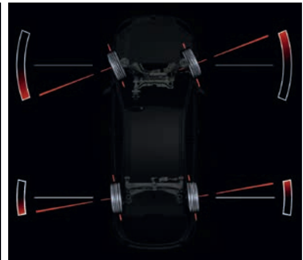
Gleichsinniges Einschlagen der Hinterachse für präzise Spurtreue bei höheren Geschwindigkeiten
