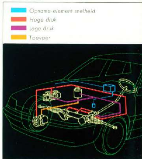
Snelheidsafhankelijke stuurbekrachtiging.
