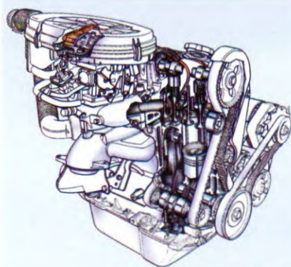
1721 cm 3 motor
