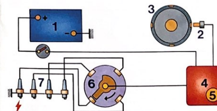
Allumage électronique intégral
