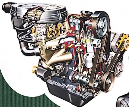
Moteur 1721 cm 3 avec boîte 5 vitesses
