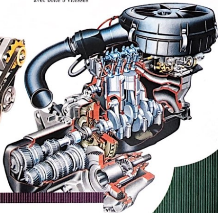
Moteur 1397 cm 3 (double corps) avec boîte 5 vitesses
