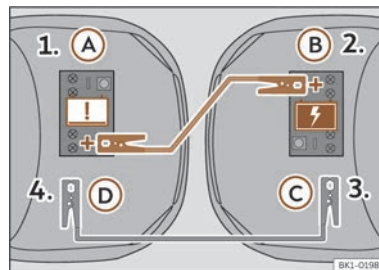
Fig. 182 Schéma de branchement des câbles de démarrage.
