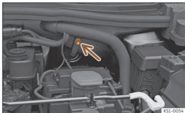
Fig. 181 Dans le compartiment avant : prise pour l'aide au démarrage (borne de mise à la terre).
