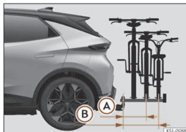
Fig. 171 Schéma de représentation de l'encorbellement maximal de la charge sur un porte-vélos pour deux ou trois vélos.
