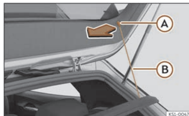
Fig. 161 Dans le coffre à bagages : démonter et remonter la plage arrière.
