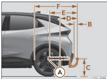
Fig. 172 Dispositif de remorquage : cotes et points de fixation.
