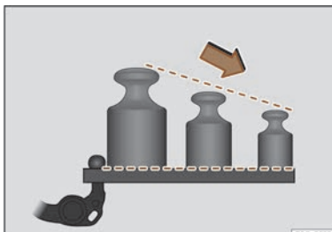
Fig. 170 Distribution recommandée du poids sur le dispositif de portage arrière.
