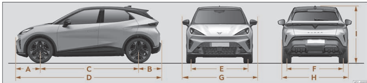
Fig. 212 Dimensions
