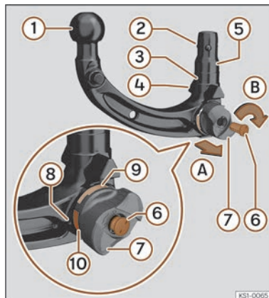
Fig. 174 Tableau général : attelage démontable pour remorque.
