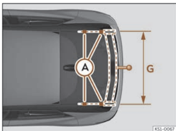
Fig. 173 Dispositif de remorquage : cotes et points de fixation.
