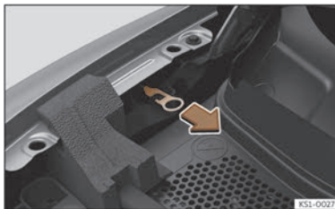
Fig. 60 Entre l'aileron droit et la charnière du capot du moteur : Poignée de déverrouillage manuel d'urgence du connecteur de charge.
