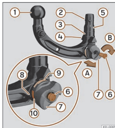
Fig. 175 Tableau général : attelage démontable pour remorque.
