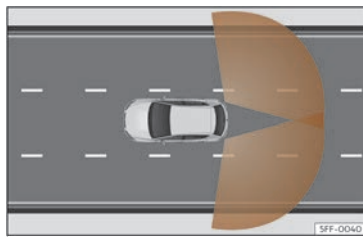
Fig. 112 Zones de détection des capteurs.
