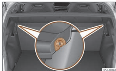
Fig. 162 Dans le coffre à bagages : démonter et remonter la plage arrière.
