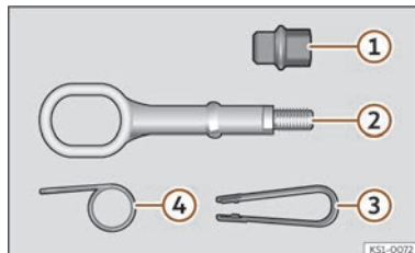
Fig. 176 Dans le coffre à bagages, sous le plancher de la surface de chargement : outillage de bord.
