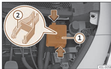
Fig. 190 Dans le compartiment avant : cache du boîtier de fusibles.
