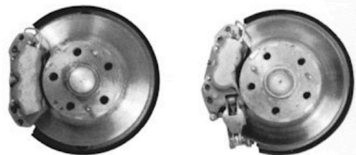
Scheibenbremsen an allen 4 Rädern mit Zweikreisbremssystem und zusätzlicher Servounterstützung
