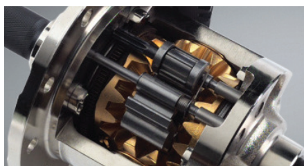
Différentiel à blocage
