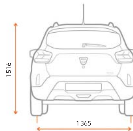
VUE ARRIÈRE
