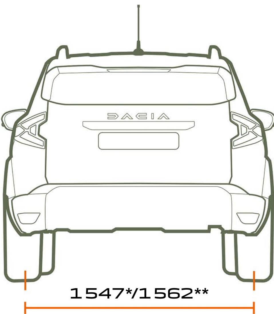
VUE ARRIÈRE
